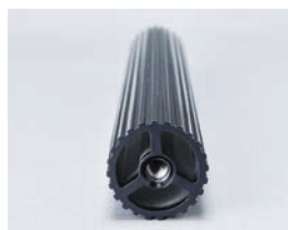
世界初の複雑形状（2重円筒形） マグネシウム材を支柱に採用。
